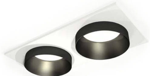
XC6525021 белый песок/черный полированный MR16 GU5.3 160x80x35 Ø150x70 (C6525, N6131)
