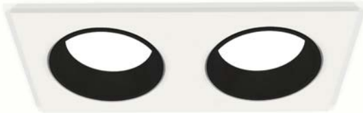
XC6525002 белый песок/черный песок MR16 GU5.3 160x80x30 Ø150x70 (C6525, N6111)
