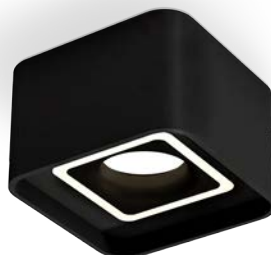
XS7833020 черный песок/черный песок MR16 GU5.3 95x95x60 (C7833, N7716)
